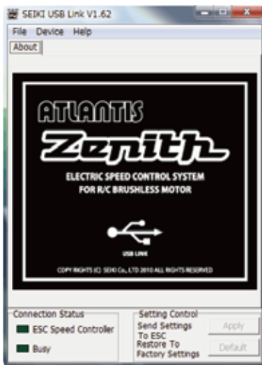
画面 1
