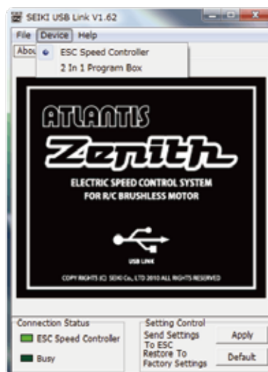
画面 2
